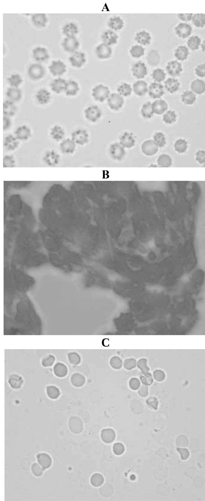
Рис. 1. Морфология эритроцитов собаки после отмывания изотоническим раствором NaCl, pH 7,4(а), после инкубации в 17,5% водном растворе ГЭК (b), после криоконсервирования и удаления криопротекторов 17,5% растворе ГЭК(с)
