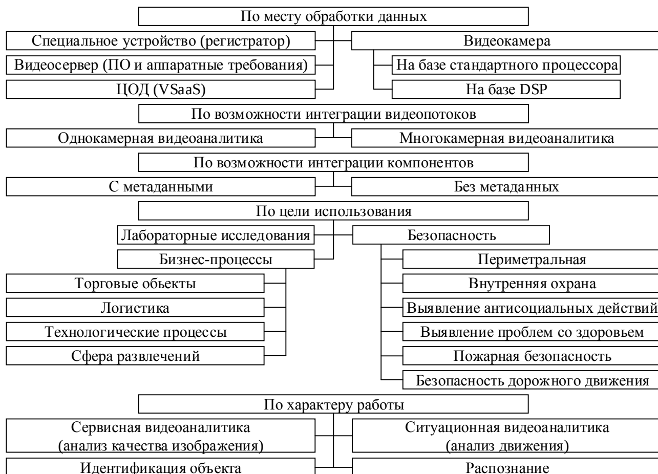
Рис. 1. Классификация видеоаналитики
