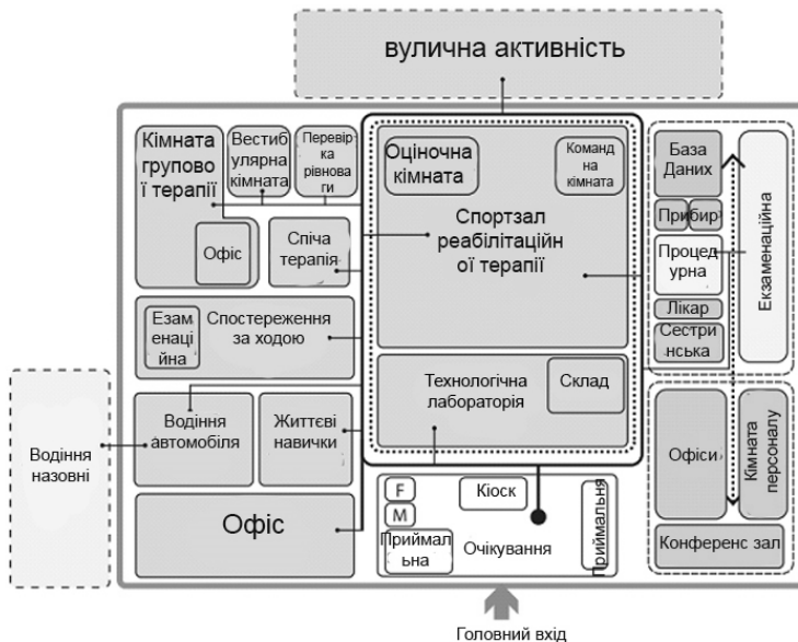
Рис. 1. Схема зонування амбулаторії реабілітаційного центру
