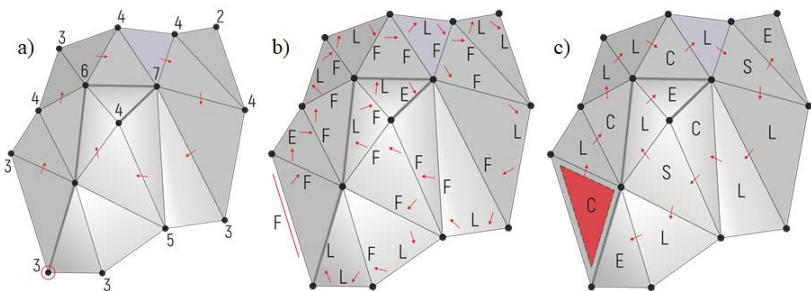
Рис. 2. Процесс кодирования выбранного участка методом а) Triangle Mesh Compression; б) Face-Fixer; в) Edgebreaker
