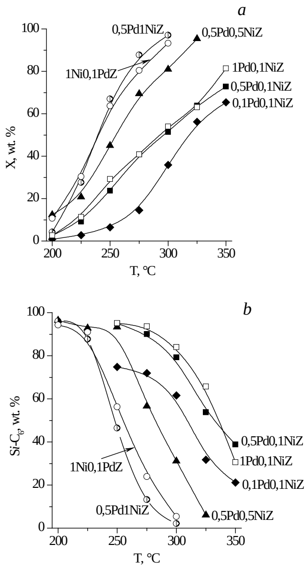
Рис. 1. Конверсія н-гексану X (а) і селективність за ізомерами гексану Si-C_6 (б) для біметалічних цеолітних каталізаторів
