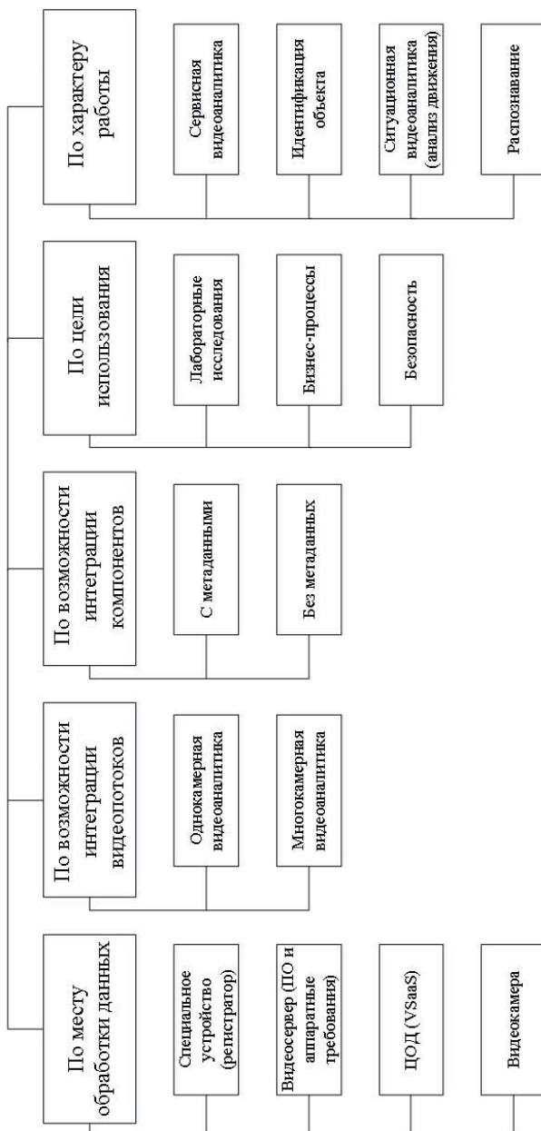
Рис. 1. Классификация видеоаналитики
