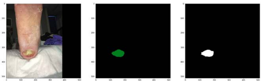
Рис. 2. Результати сегментації (2)
