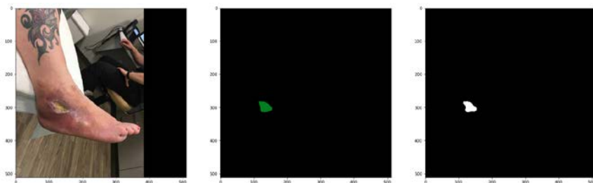
Рис. 1. Результати сегментації (1)
