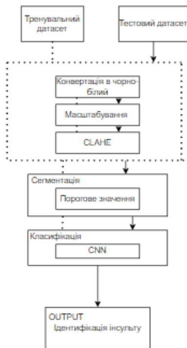
Рис. 1. Загальна архітектура
