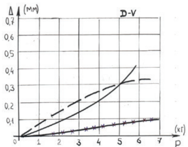
Рис. 4. Прогин препаратів цілої та синтезованої кістки у дорсо-вентральній площині: - - - ціла кістка; — пластина АО; - *-*— пластина LCP
