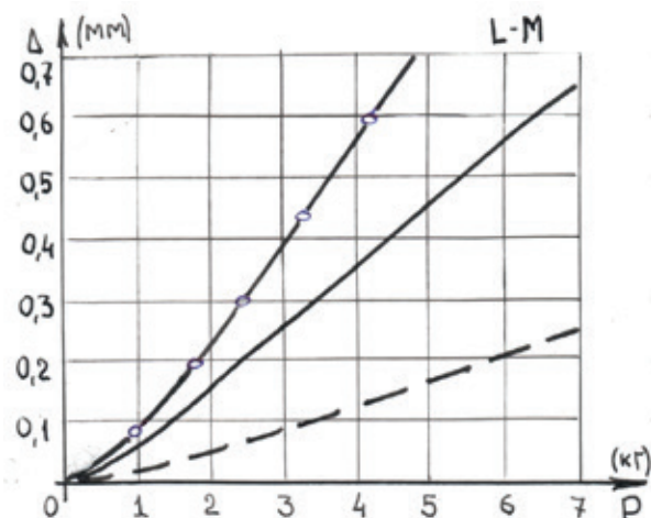
Рис. 10. Прогин препаратів цілої та синтезованої кістки у латеро-медіальній площині: - - - - ціла кістка; — пластина ДПР; -○-○- пластина Белінського
