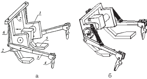
Рис. 2. Общий вид динамического лункообразователя: а – лункообразователь типа Л-2У; б – лункообразователь типа Л-2М; 1 – осто́в, 2 – навесное устройство, 3 – качающийся рычаг, 4 – игла, 5 – лыжеобразный полз, 6 – пружина
