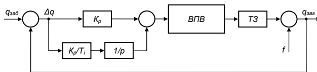
Рис. 2. Структурна схема САКПШ
