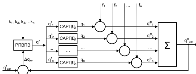
Рис. 1. Функціональна схема САКПП
