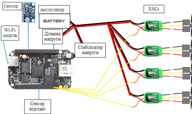
Рис. 1. Схема підключення основних елементів квадрокоптера
