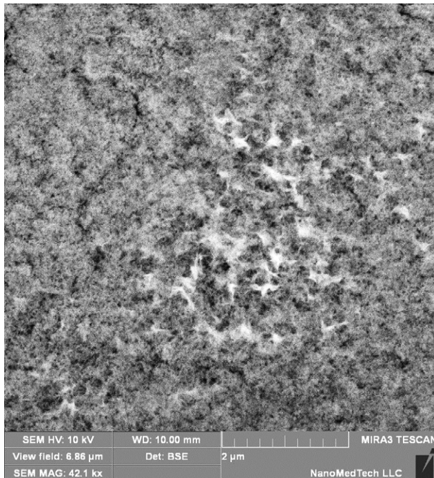
Рис. 1. Мікроснімок поверхні емалі, обробленої 0,5% водним розчином лантану азотнокислого (збільшення 42,1 тисяч разів). «Світлі» ділянки – області з підвищеним вмістом лантану
