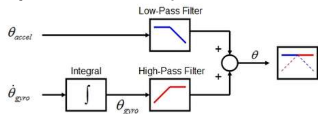
Рис. 3. Комплементарний фільтр
