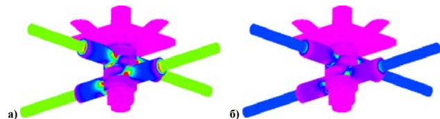
Рис. 4. Розподіл напруг по тілу вузла з'єднання: а) від руйнівного навантаження; б) від розрахункового навантаження
