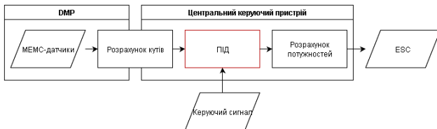
Рис. 2. Схема роботи підсистеми стабілізації
