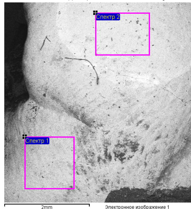
Рис. 4. Електронне зображення фрагмента поверхні емалі (збільшення в 63 рази)
