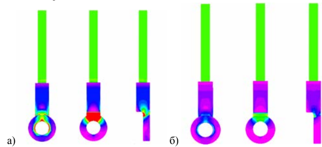
Рис. 3. Розподіл напруг по тілу наконечника: а) від руйнівного навантаження; б) від розрахункового навантаження
