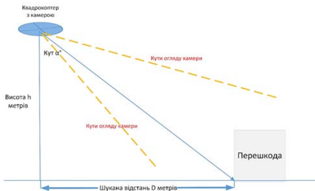
Рис. 1. Схема стереометричних обчислень
