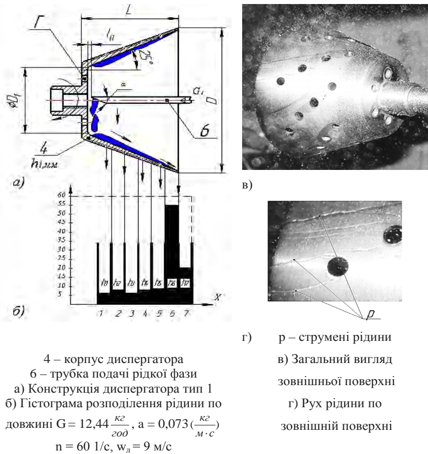
Рис. 2. Механічний диспергатор тип 1
