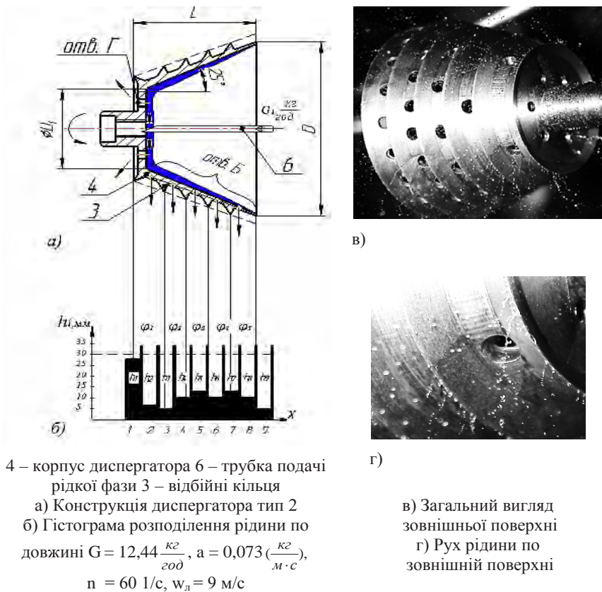
Рис. 3. Механічний диспергатор тип 2
