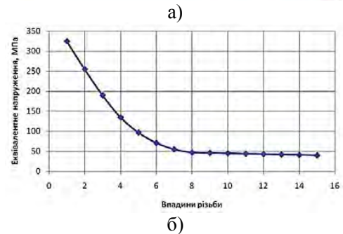
а) – у поперечному перерізі з'єднання; б) – по впадинах витків різьби ніпеля
