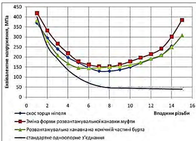
Рис. 13. Графічні залежності для трьох запропонованих варіантів зміни конструктивних елементів двоопорного замкового з'єднання та стандартного одноопорного з'єднання 3-147
