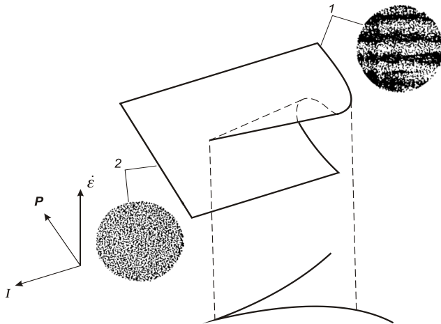
Рис. 2. Трансформация кривых течения \dot{\epsilon}(P) с ростом интенсивности вибрации I при сочетании непрерывного сдвига с ортогонально направленной к нему осцилляцией (модель «сборка»); реологические зависимости и соответствующие им структуры дисперсий: 1 – без вибрации; 2 – при вибрации с оптимальными параметрами
