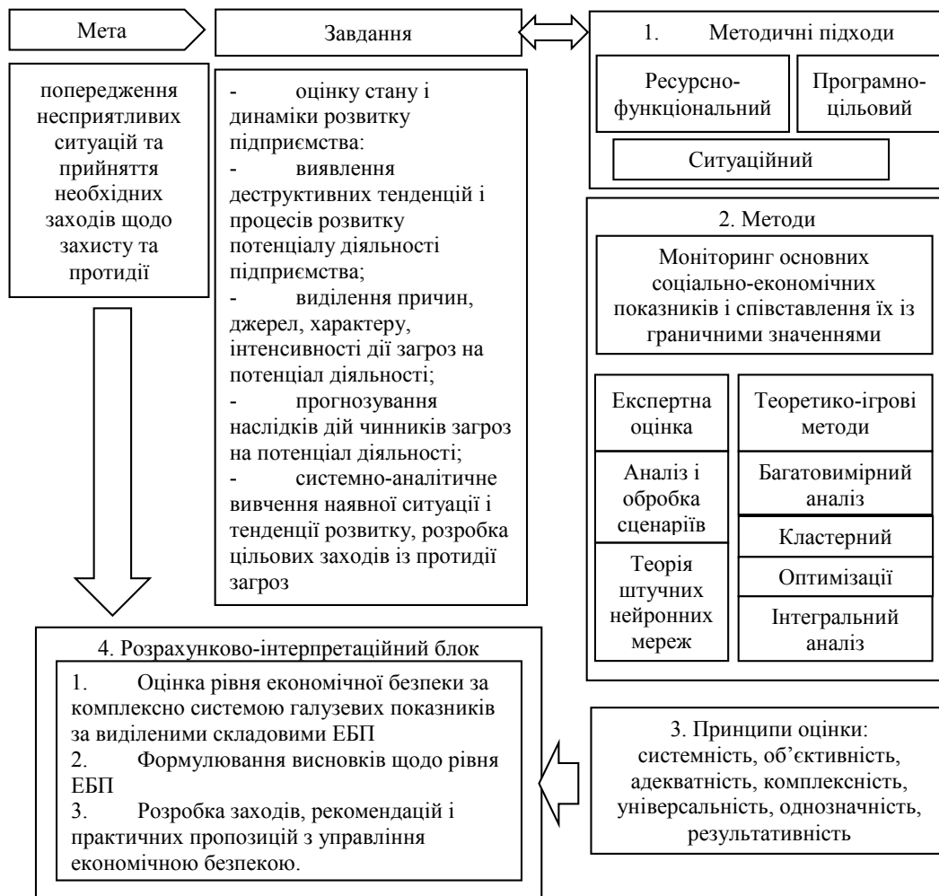
Рис. 1. Концептуальна схема оцінювання економічної безпеки підприємства
